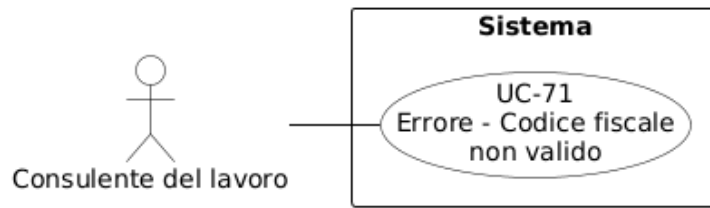
Figura 108: Diagramma del caso d'uso UC-71: Errore per codice fiscale non valido
