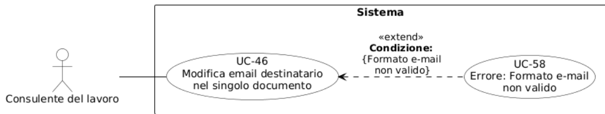
Figura 75: Diagramma del caso d'uso UC-46: Modifica email destinatario nel singolo documento
