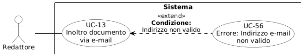
Figura 20: Diagramma del caso d'uso UC-13: Inoltro documento via e-mail
