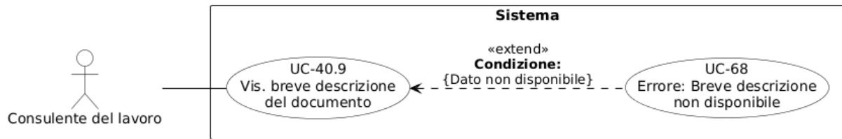
Figura 63: Diagramma del caso d'uso UC-40.9: Visualizzazione breve descrizione del documento
