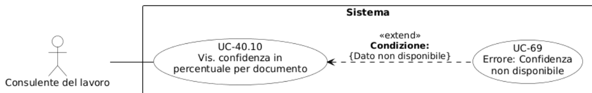
Figura 64: Diagramma del caso d'uso UC-40.10: Visualizzazione confidenza in percentuale per documento
