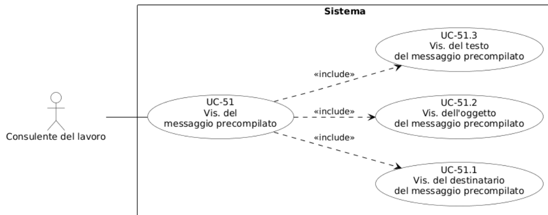
Figura 80: Diagramma del caso d'uso UC-51: Visualizzazione del messaggio precompilato
