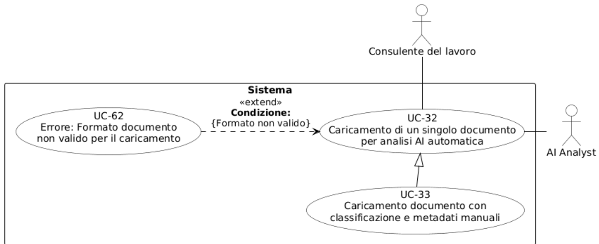
Figura 42: Diagramma del caso d'uso UC-32: Caricamento di un singolo documento per l'analisi AI automatica
