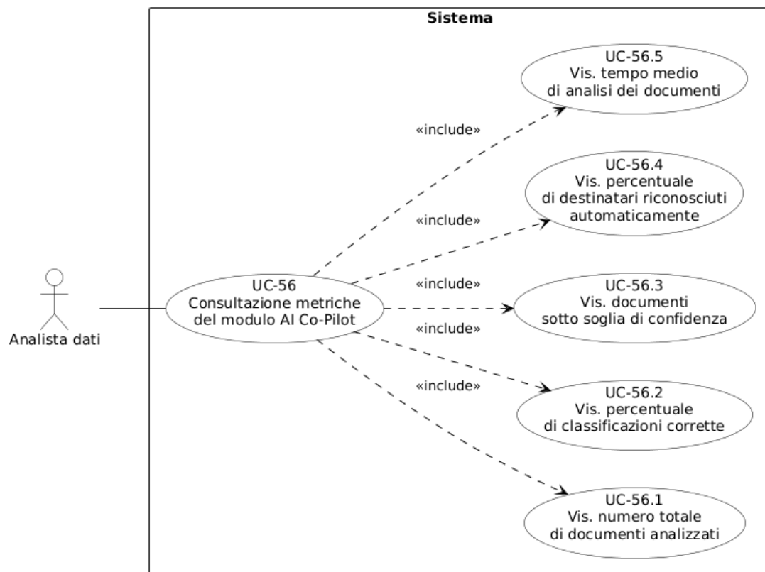
Figura 88: Diagramma del caso d'uso UC-56: Consultazione metriche del modulo AI Co-Pilot
