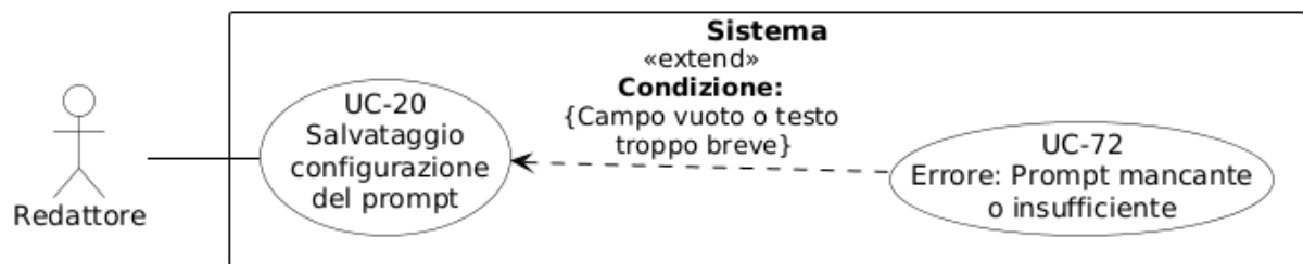
Figura 27: Diagramma del caso d'uso UC-20: Salvataggio configurazione del prompt
