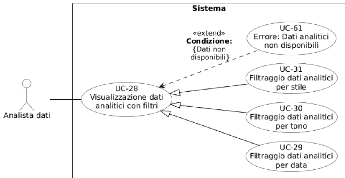
Figura 38: Diagramma del caso d'uso UC-28: Visualizzazione dati analitici con filtri
