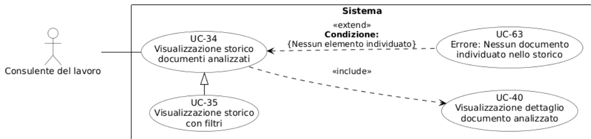
Figura 48: Diagramma del caso d'uso UC-34: Visualizzazione storico documenti analizzati
