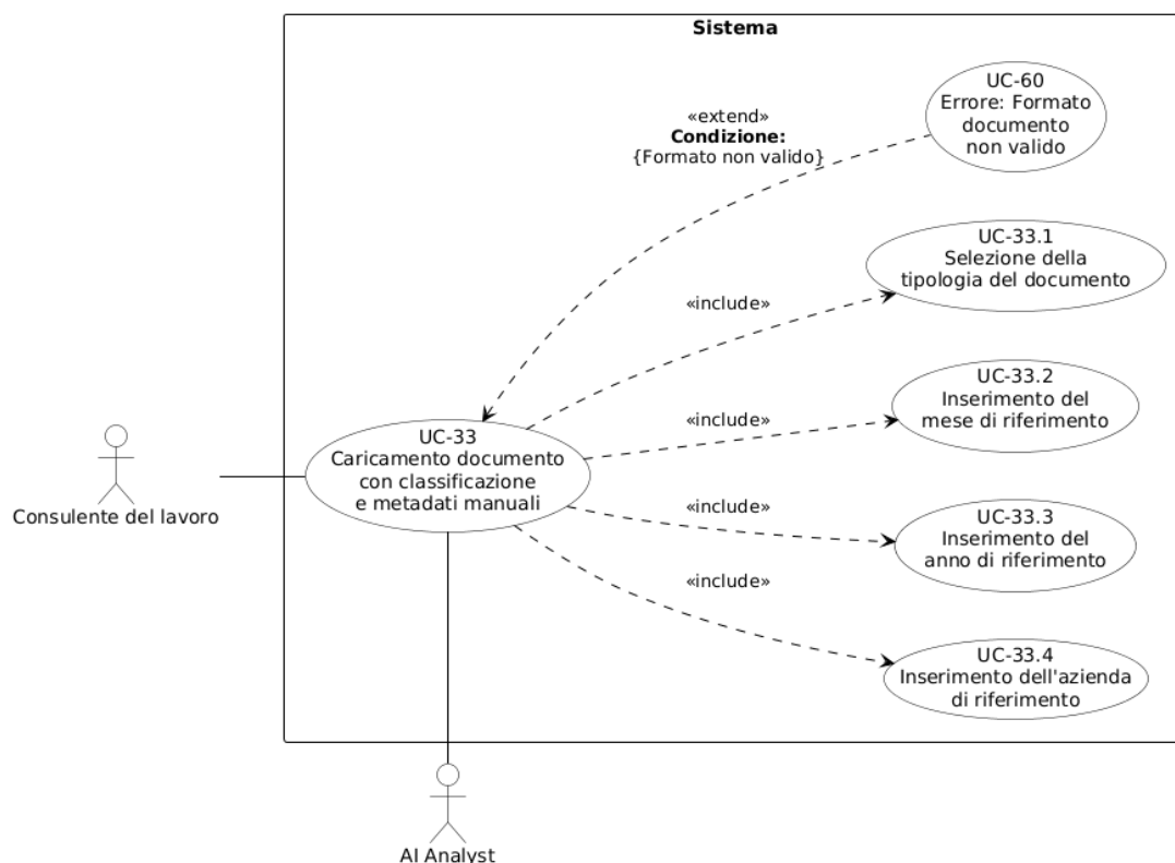
Figura 43: Diagramma del caso d'uso UC-33: Caricamento documento con classificazione e metadati manuali
