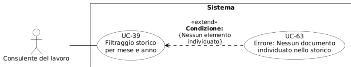
Figura 53: Diagramma del caso d'uso UC-39: Filtraggio storico per mese e anno
