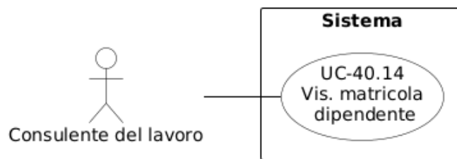
Figura 68: Diagramma del caso d'uso UC-40.14: Visualizzazione matricola dipendente
